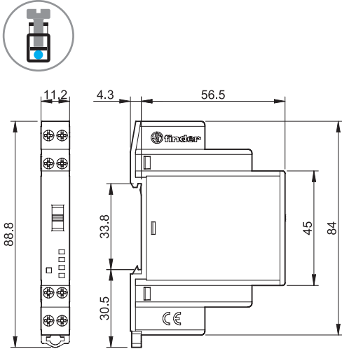
Tipo 19.21 Morsetti a vite
