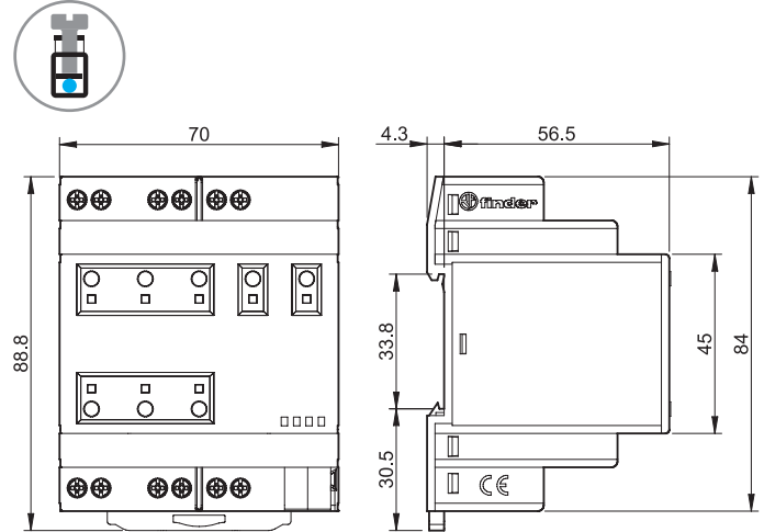
Tipo 19.6K Morsetti a vite
