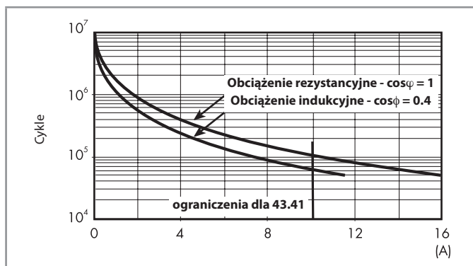
F 43 - Trwałość łączeniowa (dla AC) w funkcji prądu na zestykach
