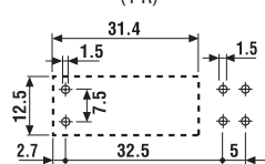
Rysunek otworów montażowych
