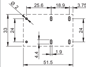
Vue coté cuivre
