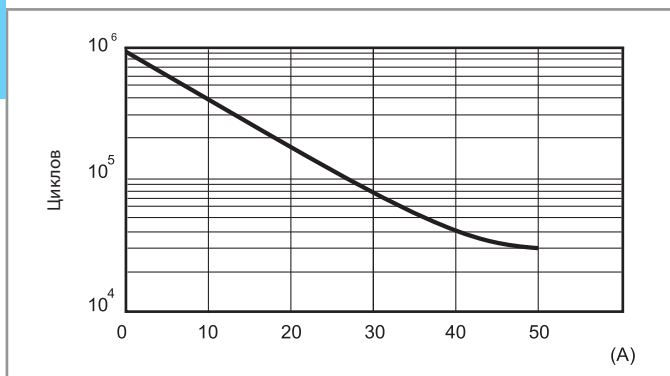
F 67 - Электрическая долговечность при ном. токе (нагрузка AC1/AC7a)
