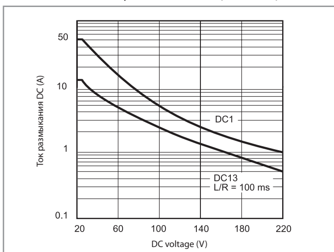
H 67 - Макс. отключающая способность DC (67.xx-x300)
