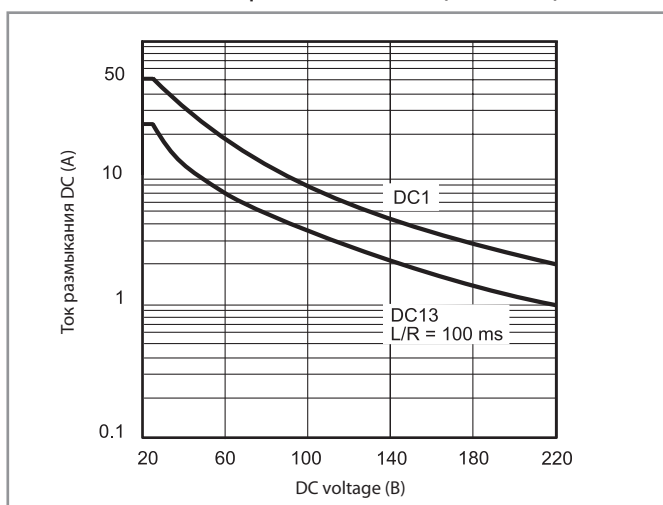
H 67 - Макс. отключающая способность DC (67.xx-x500)
