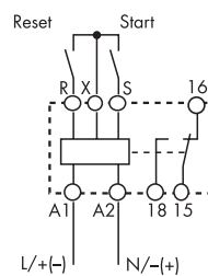
Schema di collegamento (senza START esterno)
